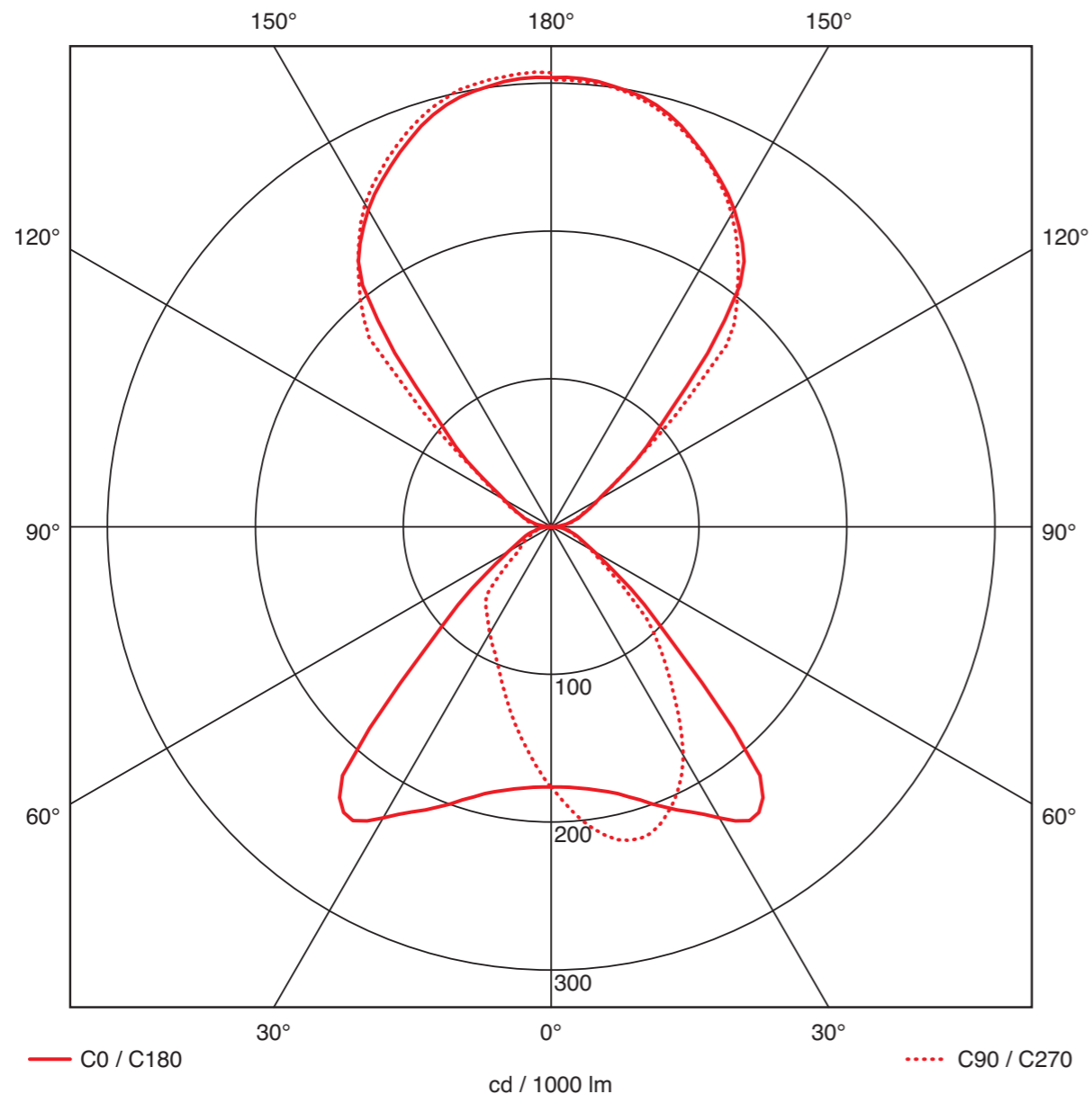
U-Fuss Lichtverteilungskurve Standard 60/40 (oben unten)
