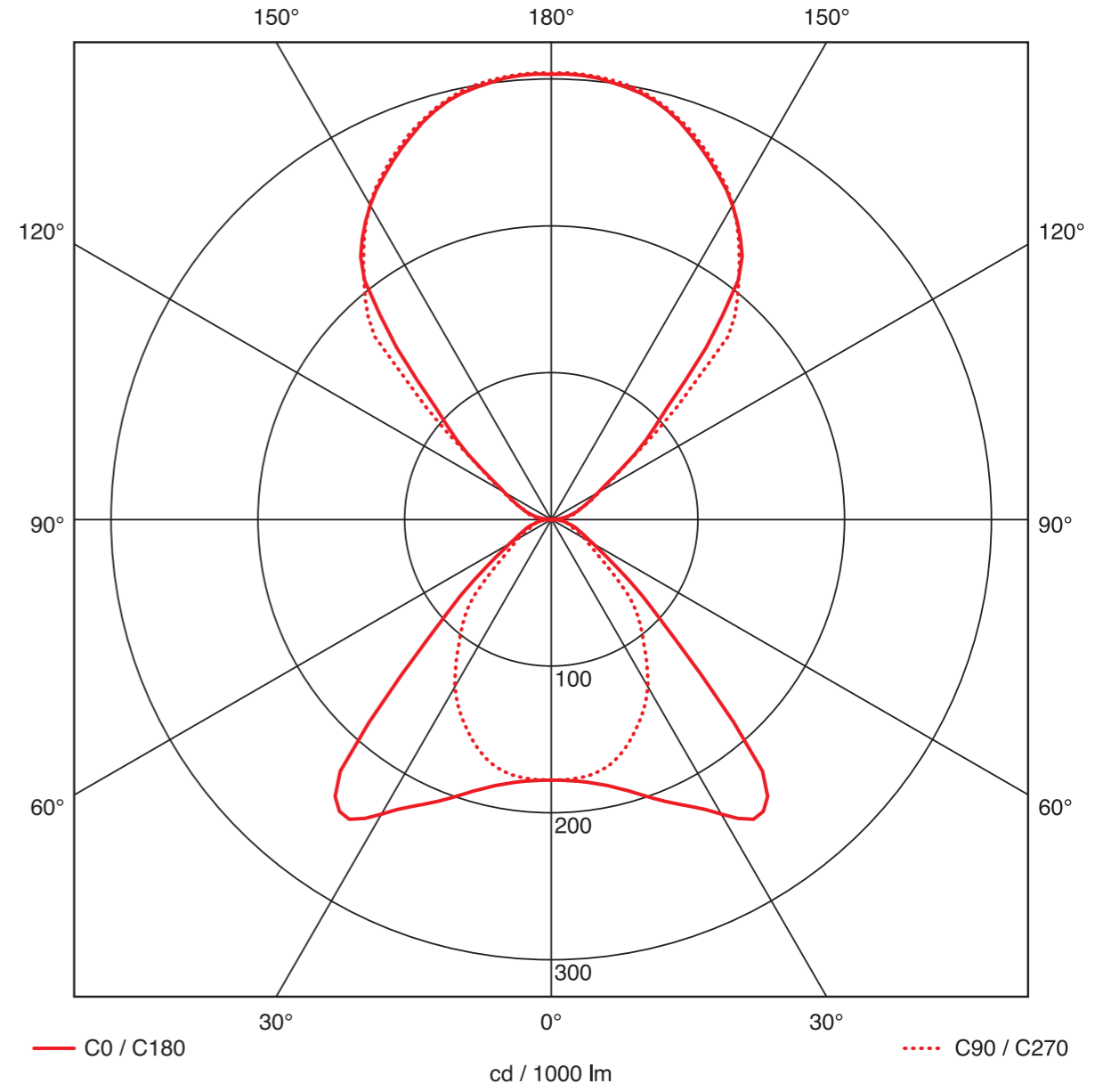
H-Fuss Lichtverteilungskurve Standard 60/40 (oben unten)
